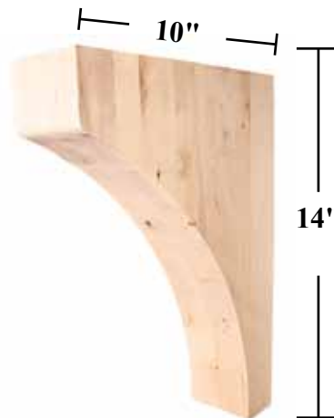
COR-T14 Specie: A, B, C, M, R 3" w x 14" h x 10" d
