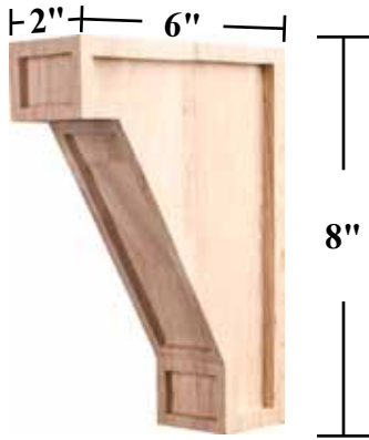
COR-MSAC8 Specie: M, R 2" w x 8" h x 6" d
