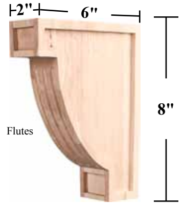
COR-FAC8 Specie: M, R 2" w x 8" h x 6" d
