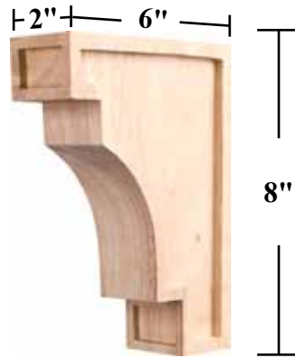
COR-CAC8 Specie: M, R 2" w x 8" h x 6" d
